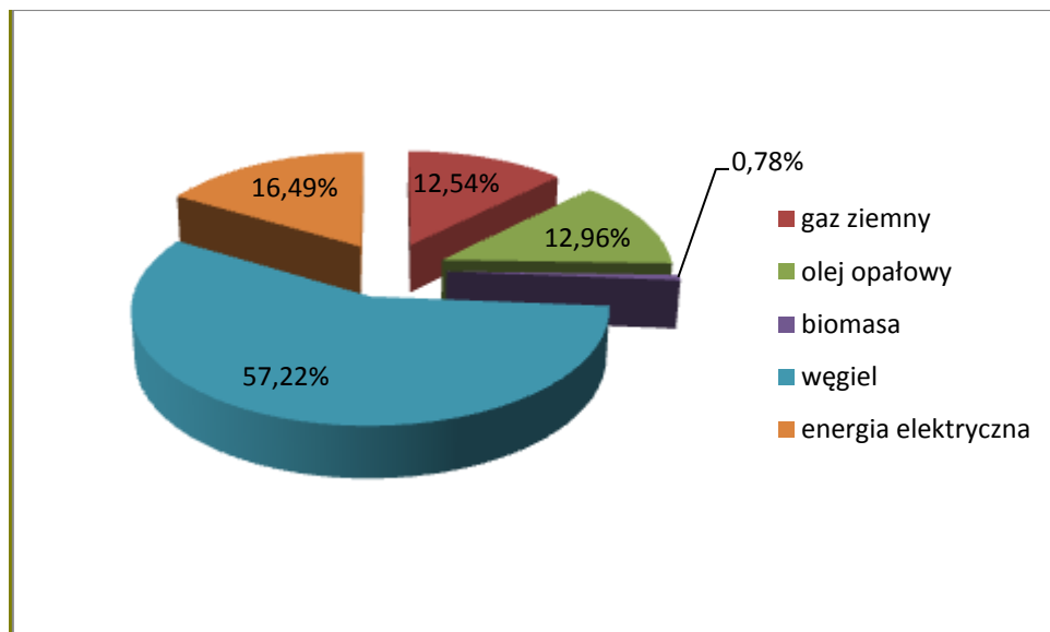
Rysunek 2-32 Struktura zużycia nośników energii w budynkach gminy Mioszów [źródło: opracowanie własne na podstawie ankietyzacji]
